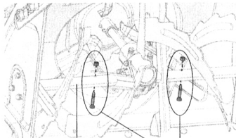
Ось шнека Предохранительный штифт
