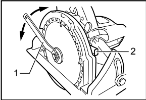
1. Llave 2. Bloqueo del eje
